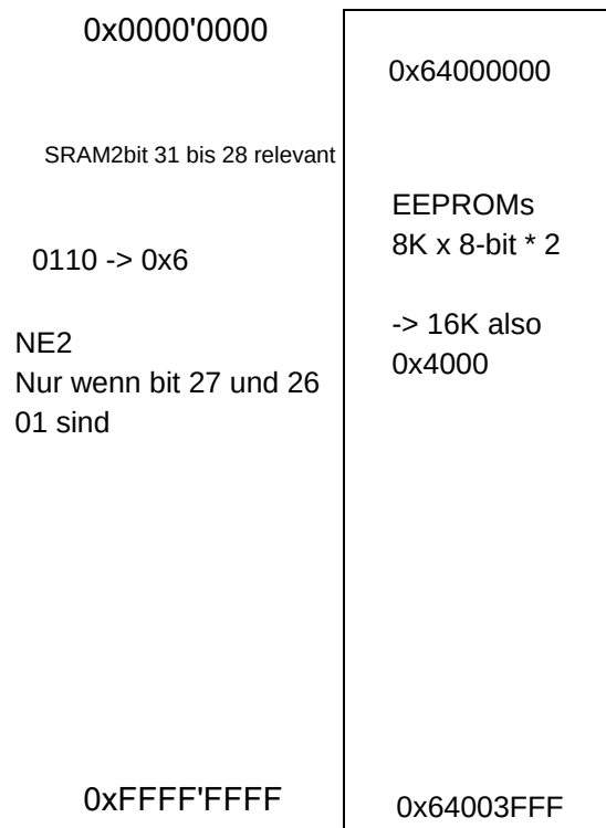
Abbildung 2: Memory Map – Speicherbereich der zwei EEPROMs
